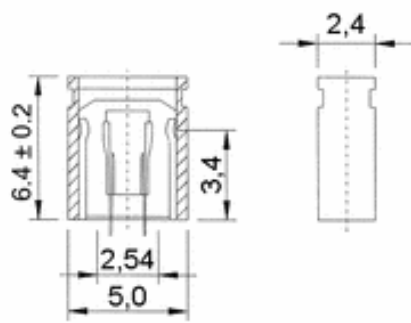
Kurzschlussbrücke, geschlossen
